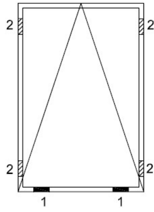
3 Kippflügel/Klappflügel
